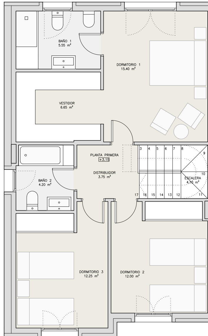
PLANTA PRIMERA Sup. construida= 77.79 m 2
