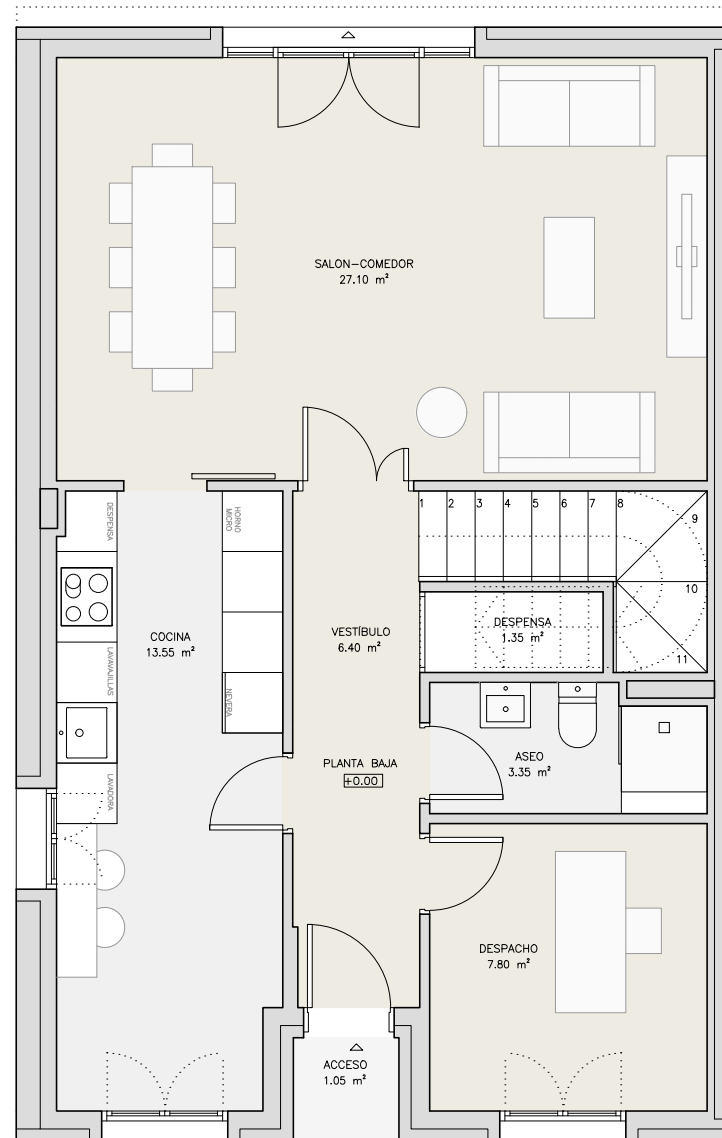
PLANTA BAJA Sup. construida= 77.90 m 2
